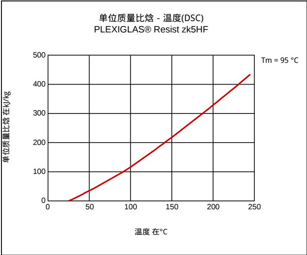
单位质量比焓 - 温度(DSC)
